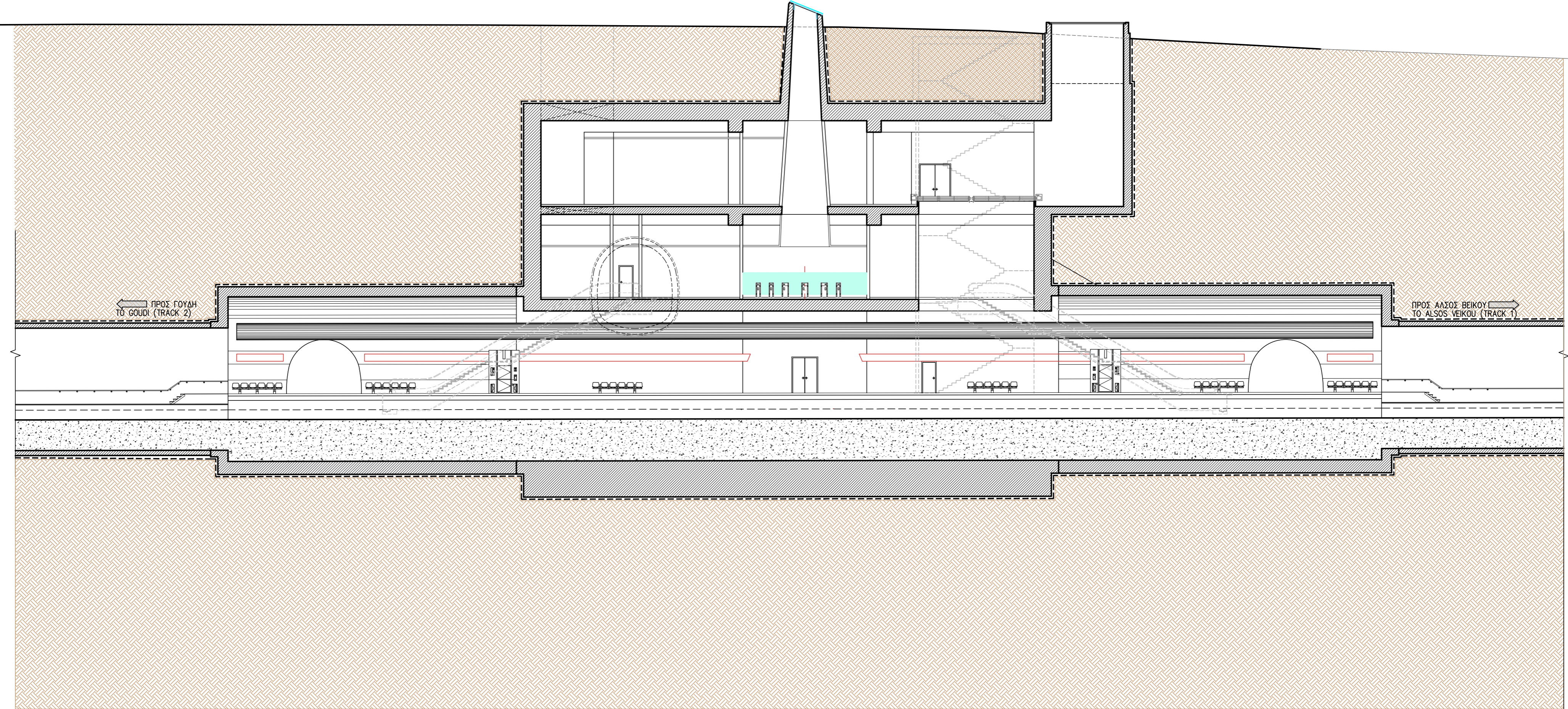
TOMH A-A
