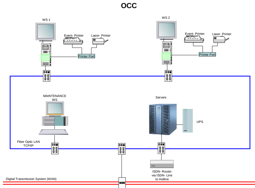
Σχήμα 2: Αρχιτεκτονική συστήματος δικτύου (ενδεικτική) ελέγχου και παρακολούθησης BACS
